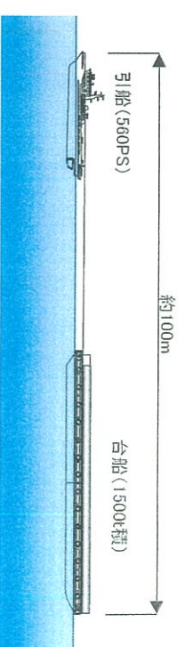
図-3 台船曳航姿図
