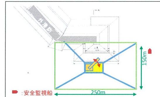
外港防波堤ブロック据付 起重機船配置計画1
