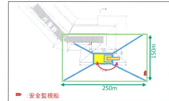
外港防波堤ブロック据付 起重機船配置計画2
