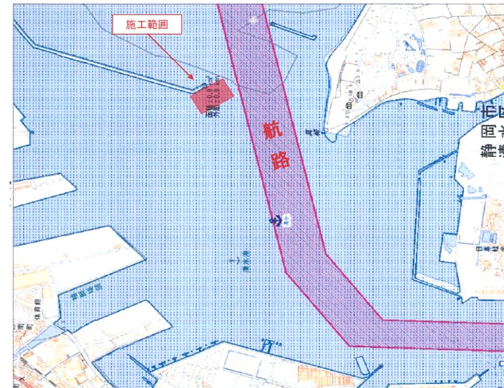
清水港 航路及び据付作業位置図
