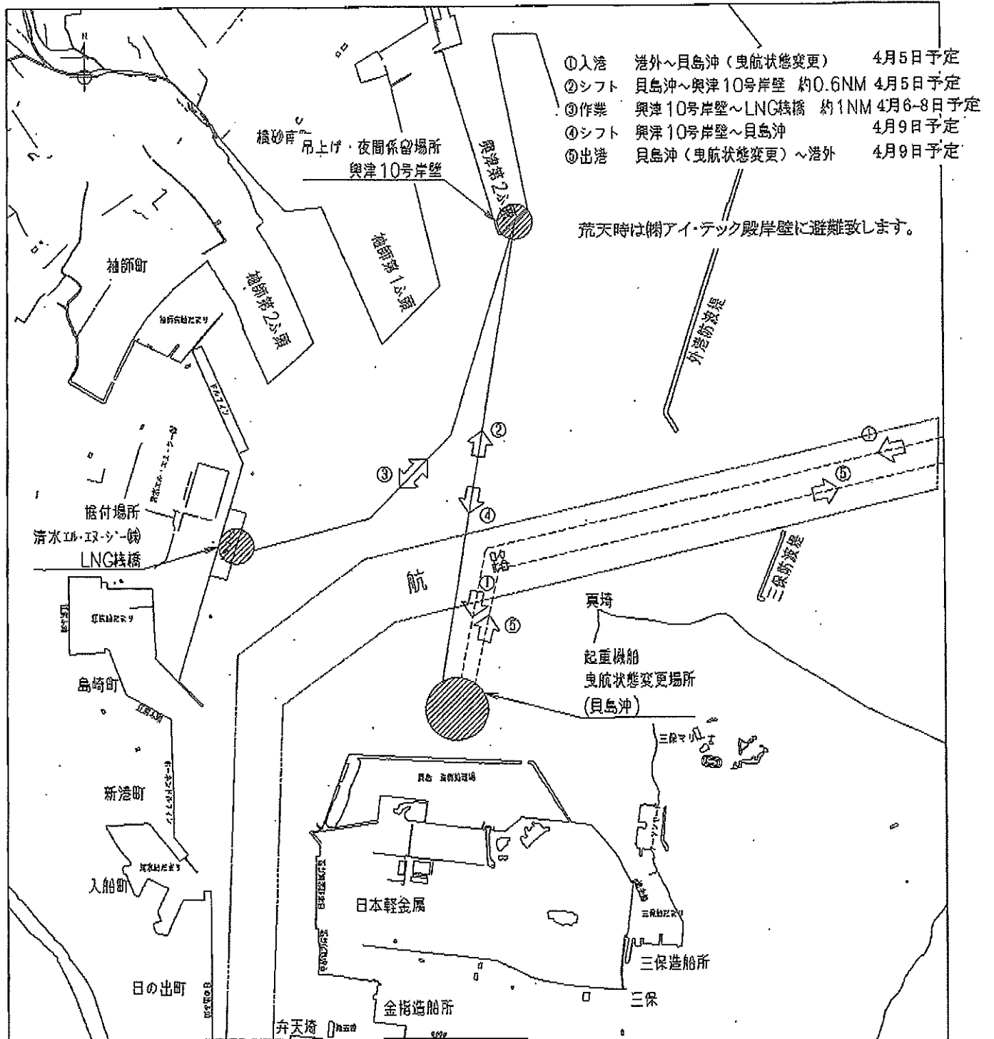
600t吊起重機船「宏栄号」曳航経路図(加内良助氏) S=1/2000
