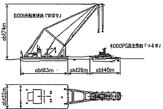
600t吊起重機船「宏栄号」曳船図(横断) 1/2000
