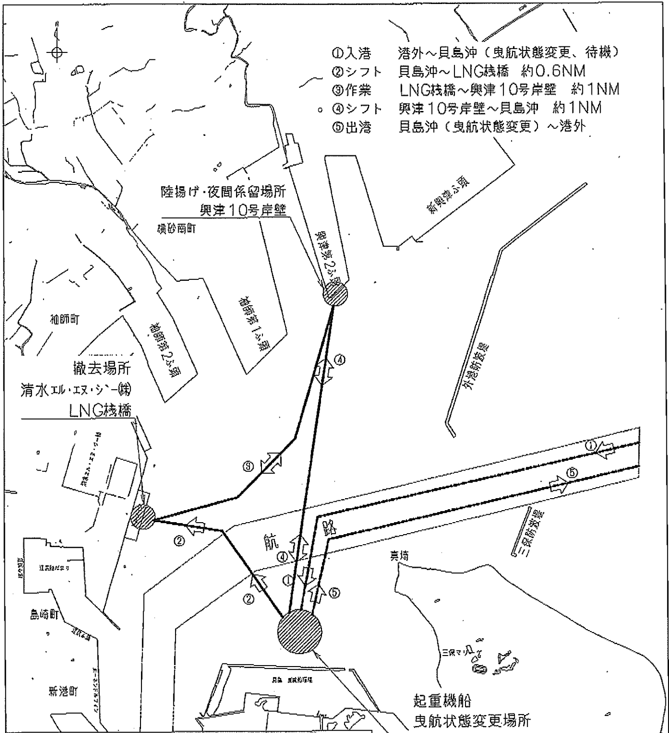
600t吊起重機船「宏栄号」曳船図(横断) 1/2000
