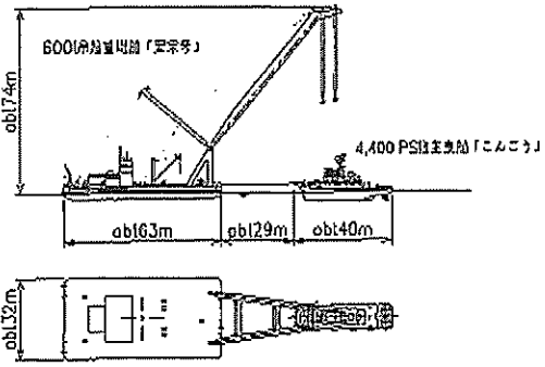
600t吊起重機船「宏栄号」曳航経路図 (清水港内)
