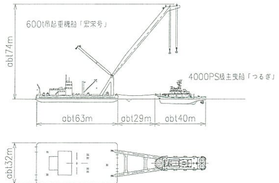
600t吊起重機船「宏栄号」曳航要領図【港内曳航時】 S=1/2000
