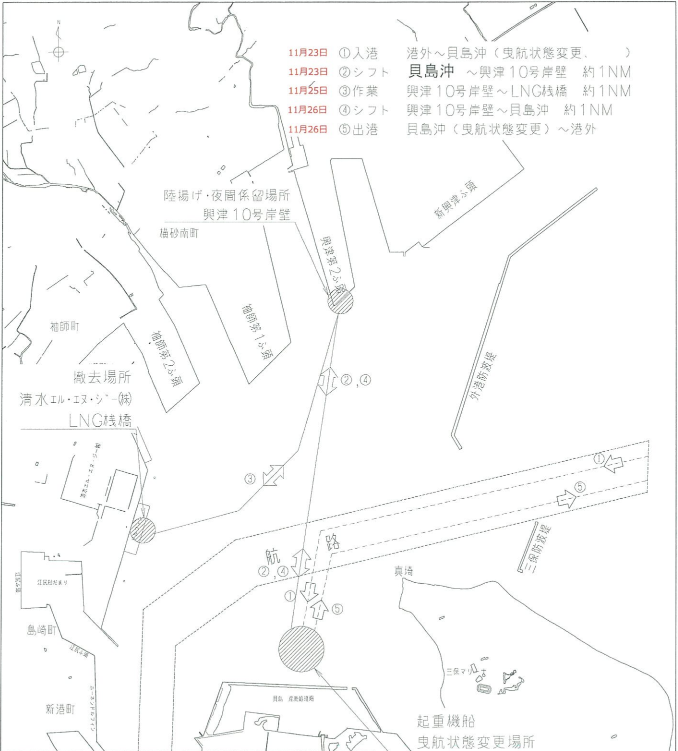
600t吊起重機船「宏栄号」曳航要領図【港内曳航時】 S=1/2000
