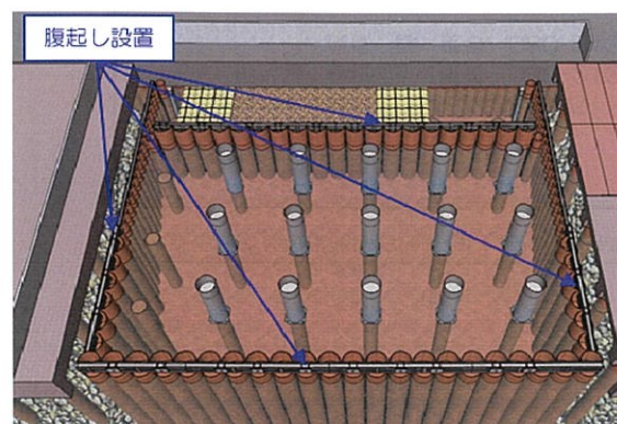
③腹起し設置
