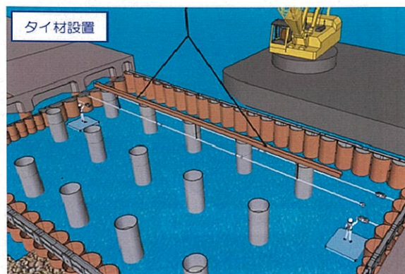
④タイ材設置
