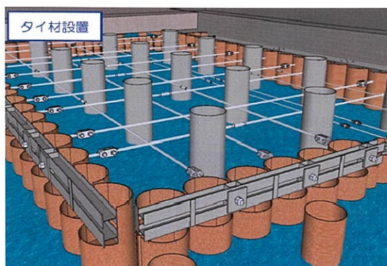
④タイ材設置
