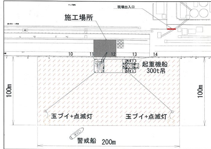
施工箇所及び夜間停泊場所(富士見埠頭4号岸壁)
