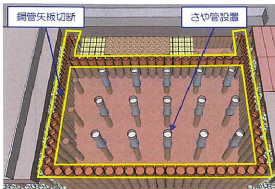
②鋼管矢板切断・さや管設置
