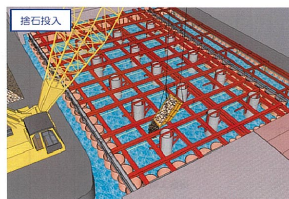
⑤捨石投入
