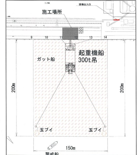
施工箇所及び夜間停泊場所(富士見埠頭4号岸壁)
