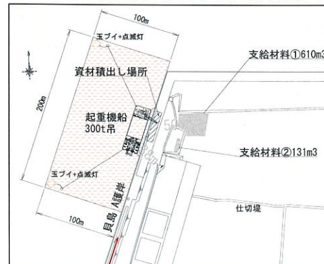
施工箇所及び夜間停泊場所(貝島地区)
