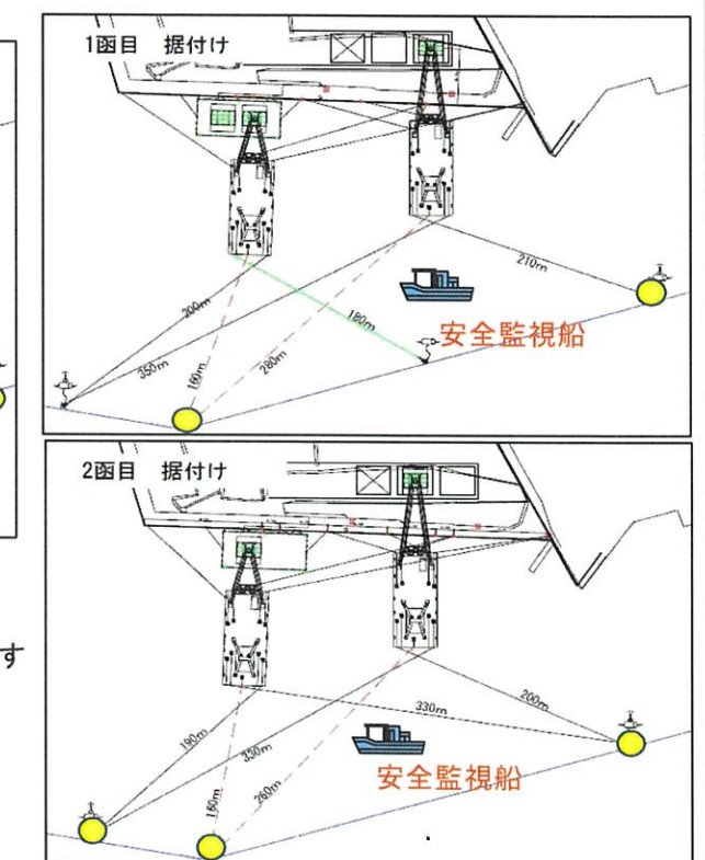
④ 鋼殻据付平面図(清水港 貝島地区)
