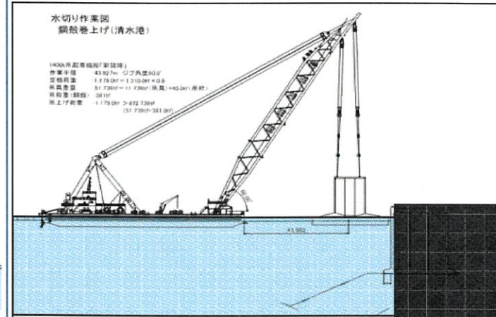
施工要領図
