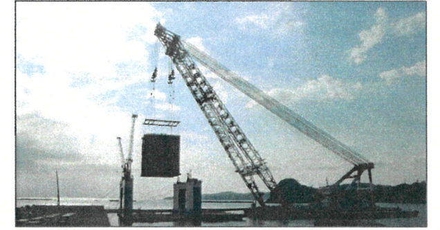
① 鋼殻吊込み(津松坂港)
