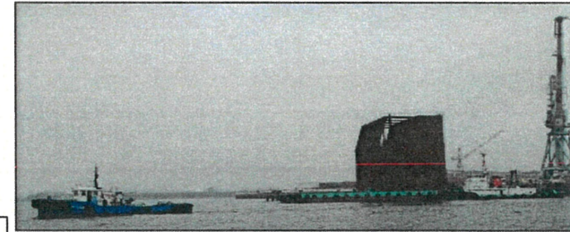
② 本体工 鋼殻海上運搬(津松坂港→清水港)
