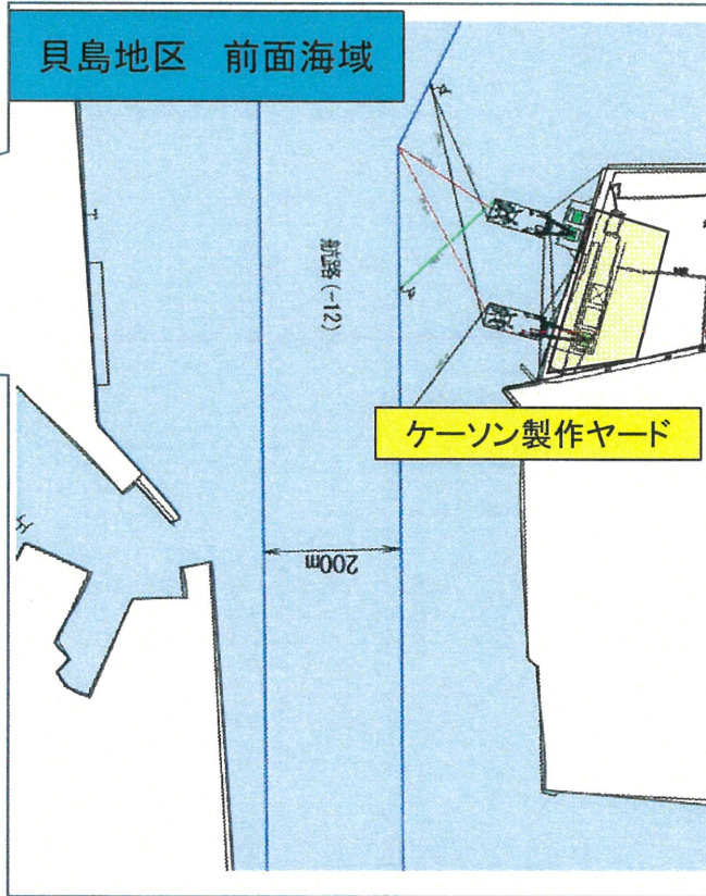
施工要領図
