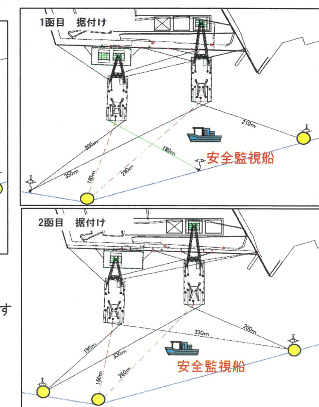
④ 鋼殻据付平面図(清水港 貝島地区)
