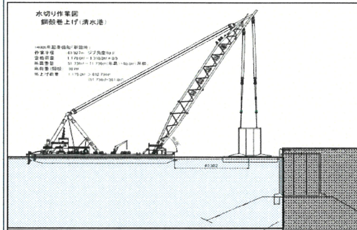
施工要領図
