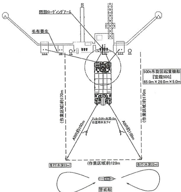
(図-3) 係留要領図(ENEOSシーハースNo.1)
