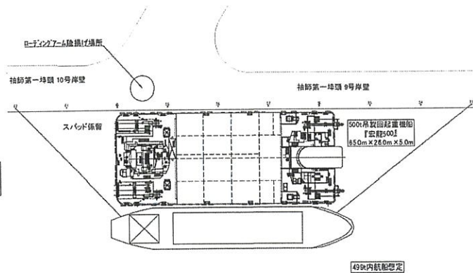
(図-4) 係留要領図(袖師第一埠頭)
